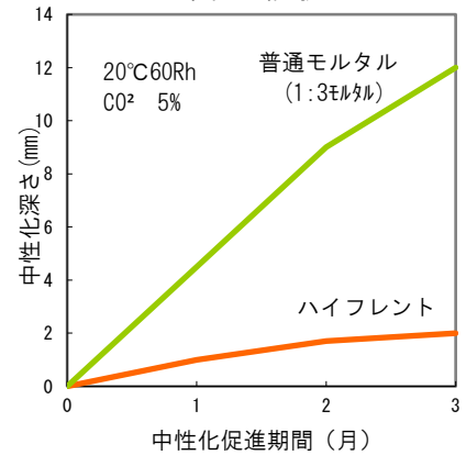
中性化試験
